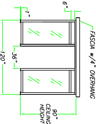
ELEVATION A
