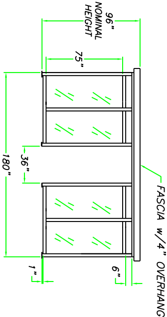
ELEVATION A
