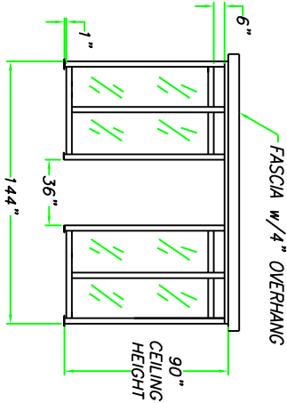
ELEVATION A
