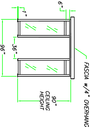
ELEVATION A
