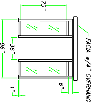
ELEVATION A
