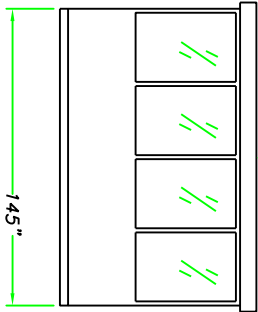
ELEVATION B
