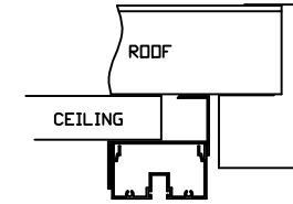
VIEW A-A
